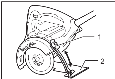
► 1. Clamping nut 2. Base
