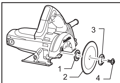
► 1. Brida interior 2. Disco de diamante 3. Brida exterior 4. Tornillo hexagonal
