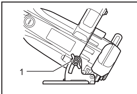
► 1. Clamping nut
