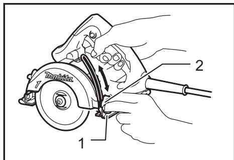
► 1. Base 2. Tuerca de fijación
